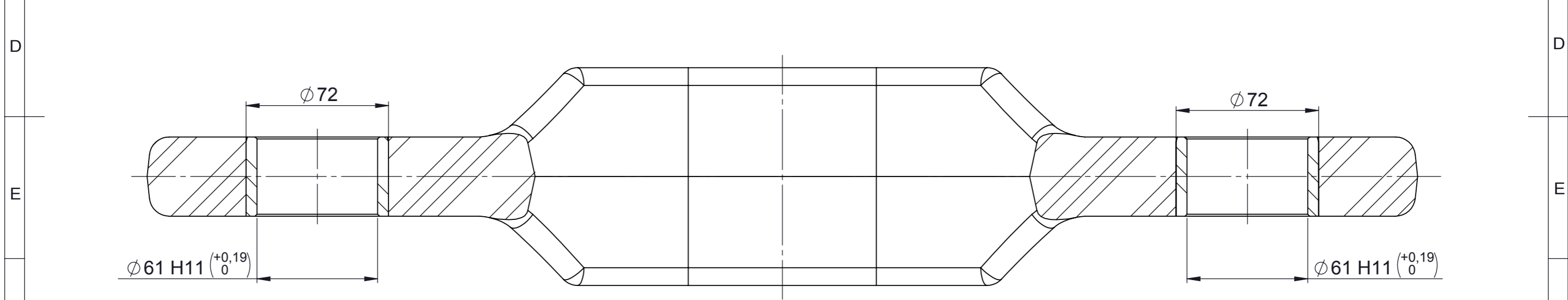
PRESEK A-A RAZMERA 1 : 2
