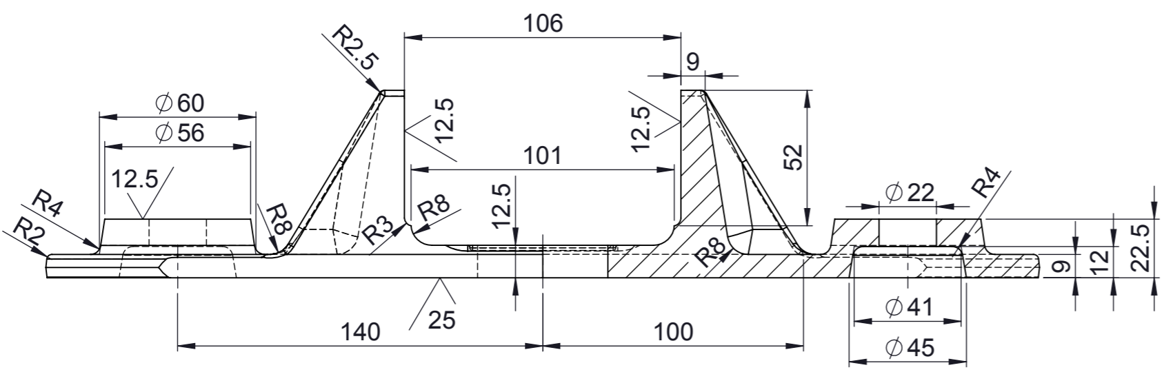
PRESEK A-A
